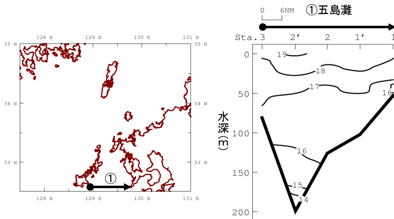
図1 水温鉛直断面図
